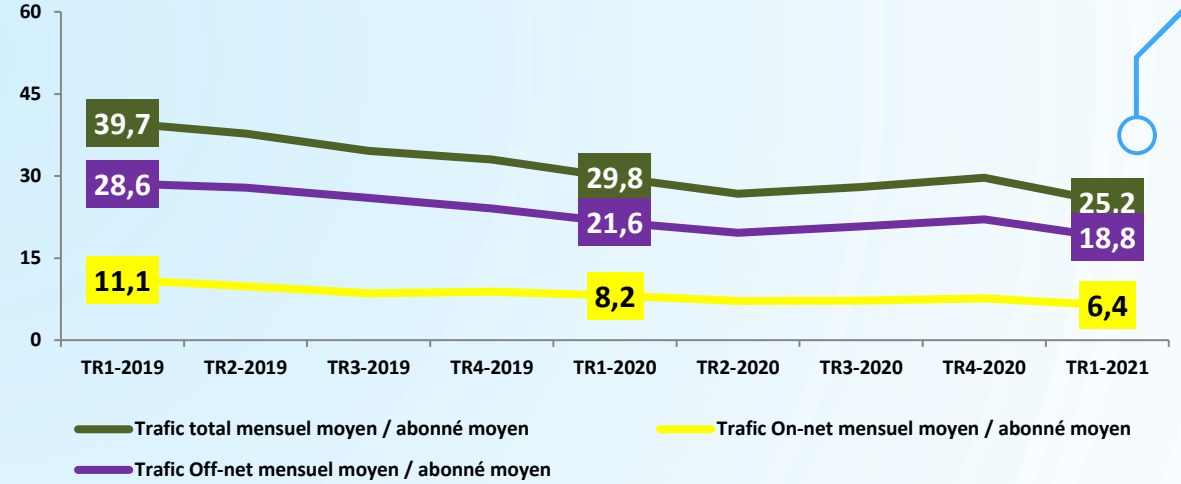
Evolution du trafic voix fixe national mensuel moyen par abonnement
