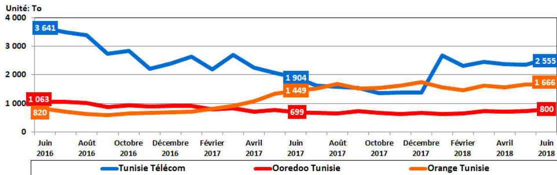
Fig18 : Evolution du trafic data mobile des clés 3G/4G par opérateur 3 .
